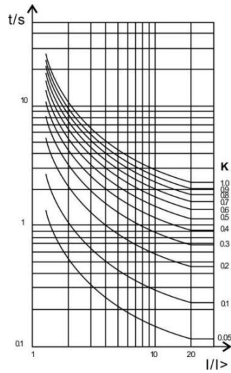
IDMT Normal Inverse
